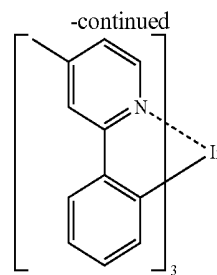
Ir(mppy) 3
