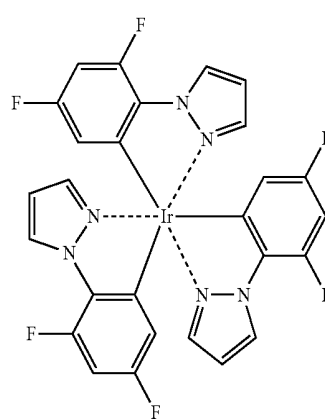
Ir(dfppz) 3
